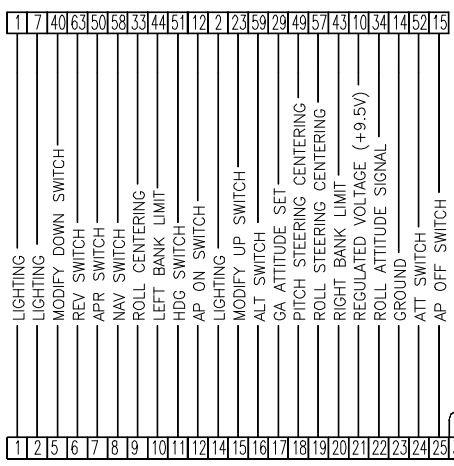
(CD 168) PROGRAMMER
