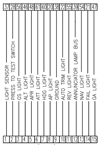
(CD 171) ANNUNCIATOR
